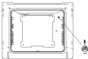
Oświetlenie piekarnika
