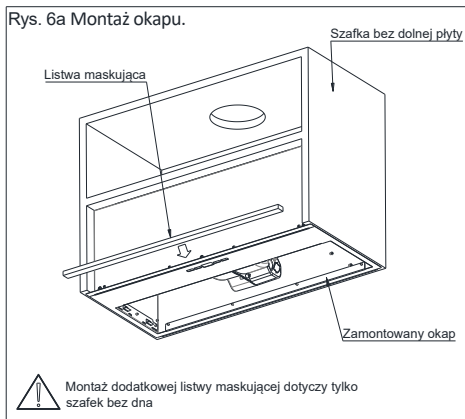
Rys. 6a Montaż okapu.
