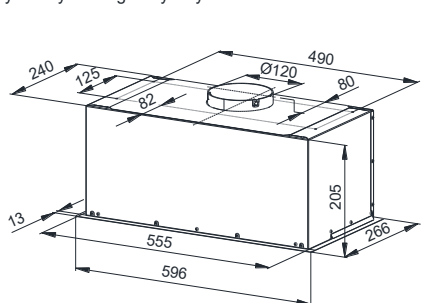
Rys. 2 Rysunek gabarytowy
