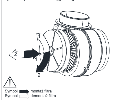
Rys. 7 Wymiana filtra węglowego.
