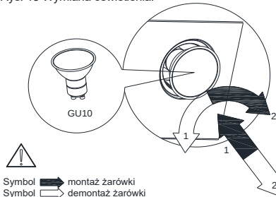
Rys. 13 Wymiana oświetlenia.
