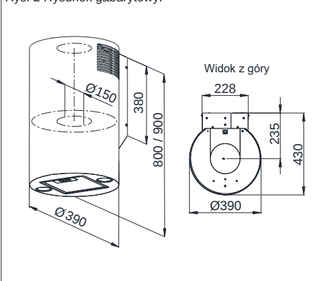
Rys. 2 Rysunek gabarytowy.
