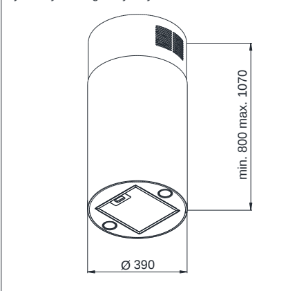
Rys. 2 Rysunek gabarytowy.
