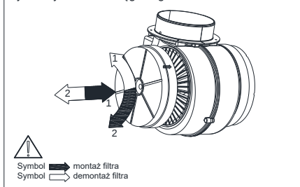
Rys. 9 Wymiana filtra węglowego.
