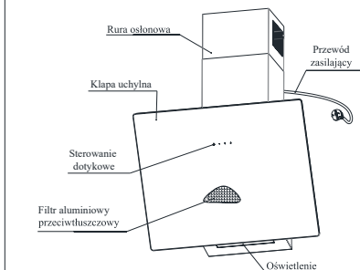
Rys. 1 Rysunek poglądowy okapu kuchennego.
