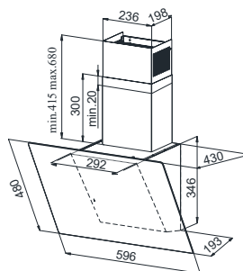
Rys. 2 Rysunek gabarytowy.
