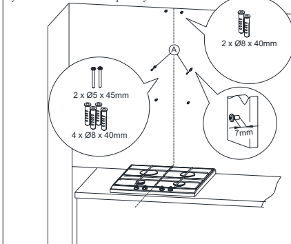
Rys. 7 Zawieszenie okapu.
