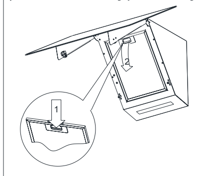
Rys. 8 Ustawienie okapu kuchennego.
